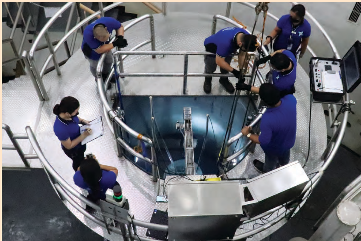
Идет загрузка топливного стержня в активную зону филиппинской подкритической сборки в учебных и исследовательских целях (SATER) на Филиппинах. (Фотография предоставлена Филиппинским институтом ядерных исследований (ФИЯИ))
