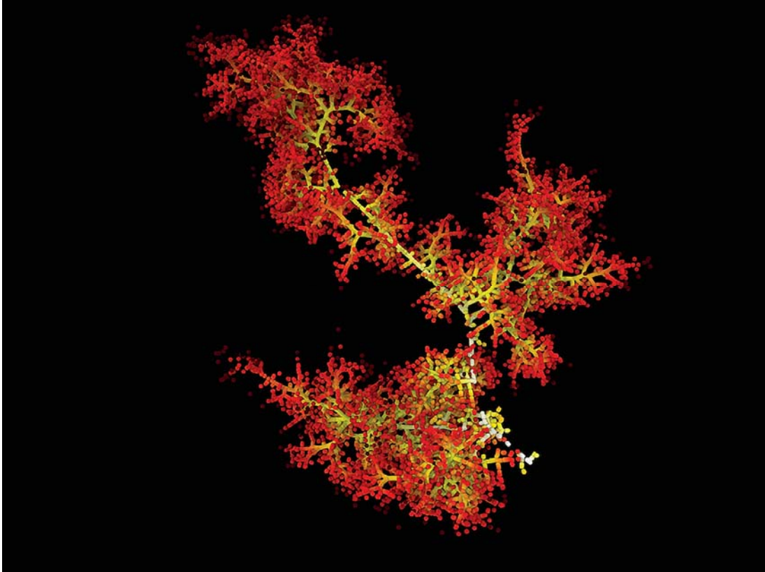
الشكل ١ - تمثيل لمحاكاة الديناميات الجزيئية للأضرار اللاحقة بجدار المفاعل الاندماجي مُقَدَّم من معهد ماكس بلانك لفيزياء البلازما الكائن في ألمانيا. (صورة مستنسخة مهداة من معهد ماكس بلانك لفيزياء البلازما، ألمانيا)
