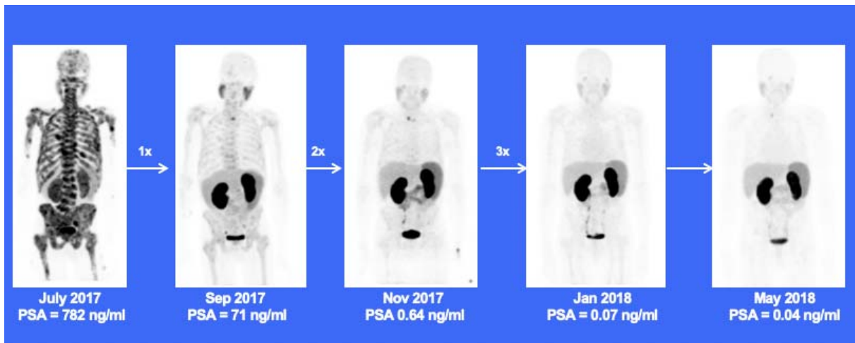
الشكل ١ - النتائج التي عرضها المشاركون في الاجتماع التقني بشأن إمدادات الأكتينيوم-٢٢٥، ويتضح منها نجاح استخدام المستحضر البروستاتي الغشائي المحتوي على الأكتينيوم-٢٢٥ (Ac-225-PSMA) في علاج سرطان البروستاتا.
