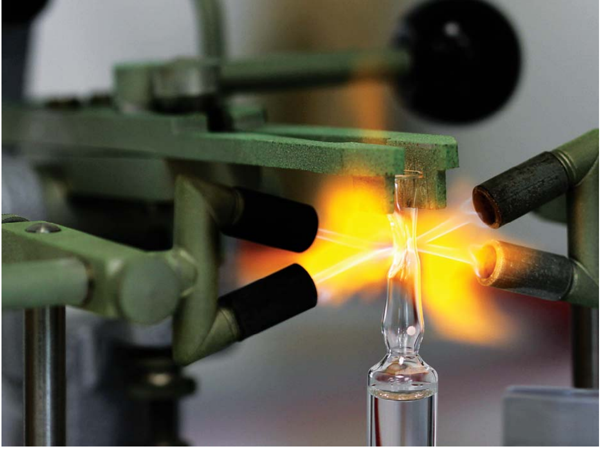
الشكل ١ - ختم المواد المرجعية للكربونات الصادرة عن الوكالة، وهي أحد المعايير الضرورية لمعايرة ورصد النظائر المستقرة لثاني أكسيد الكربون بدقة عالية.
