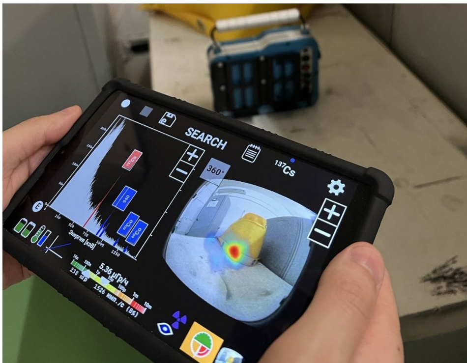
南乌克兰核电厂正在使用的γ射线成像光谱仪。这一设备由原子能机构利用英国提供的预算外捐款采购，并于2023年5月26日交付给南乌克兰核电厂。
