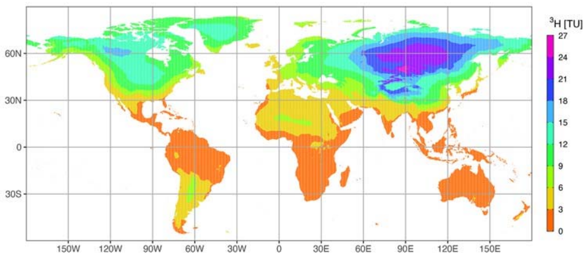
Fig. 8. Niveles actuales de tritio en la precipitación. La sigla TU se refiere a la actividad de tritio expresada en unidades de tritio.
