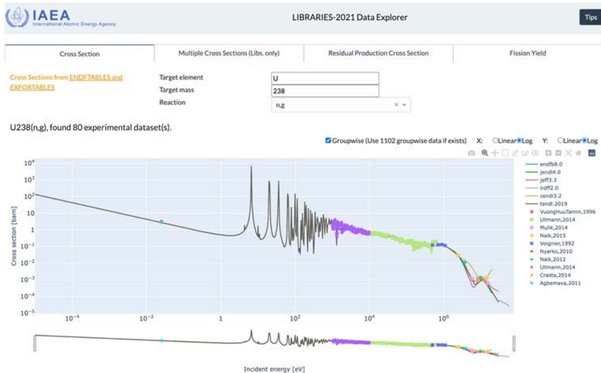
Fig. 1. El Buscador de Datos de Libraries-2021 para la recuperación y la representación de datos sobre reacciones nucleares, utilizando como ejemplo la reacción de captura de neutrones de uranio 238.
