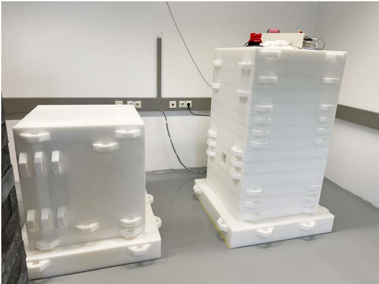
Fig. 4. Ensamblaje de blindaje en el que se encuentra el generador de neutrones de deuterio-deuterio durante su fase de puesta en servicio.
