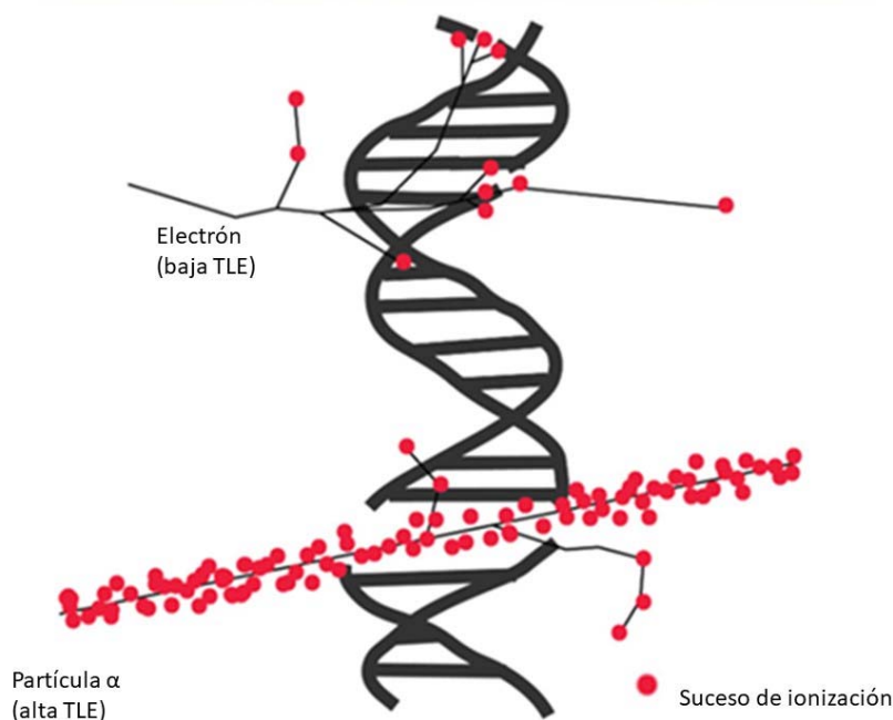
Fig. 12. Comparación del efecto de las partículas alfa y beta en el ADN diana. (Fotografía cortesía del Departamento de Energía de los Estados Unidos)
