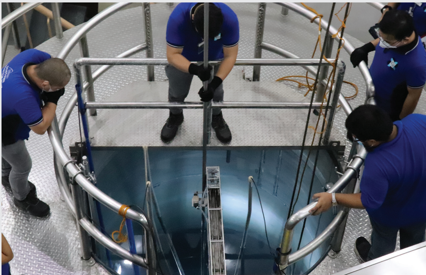
Топливный стержень загружается в активную зону подкритической сборки. (Фото: ФИЯИ)
