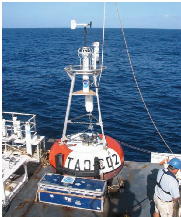
海洋酸化的趋势在大洋中正在得到检测
